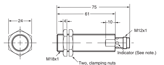
E2A-S18LS08-M1-□
