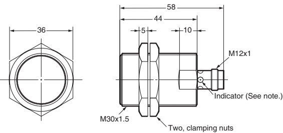
E2A-S30KS15-M1-□
