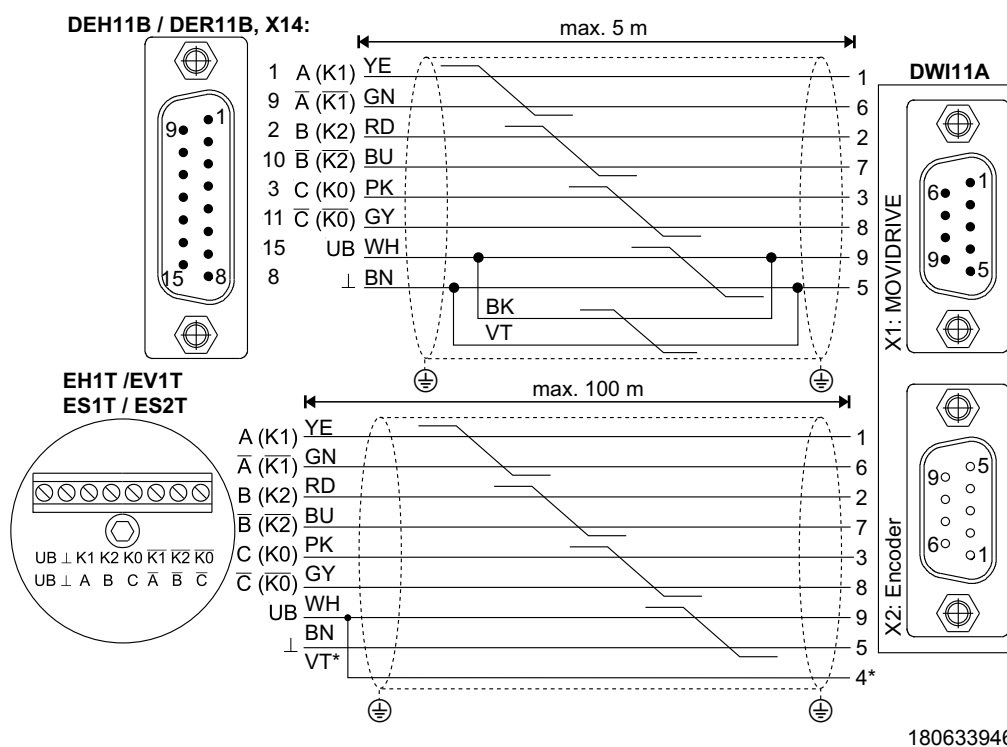
Figura 15: Conectar el encoder TTL EV1T como encoder externo a MDX a través de DWI11A
