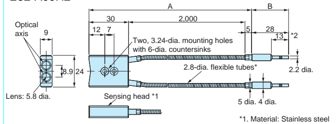
E32-A09H2
