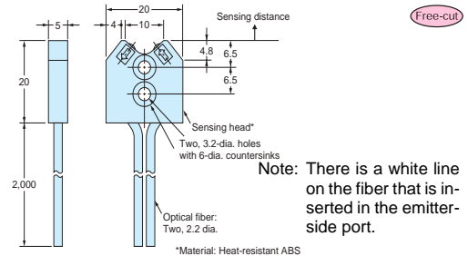
E32-L25A
