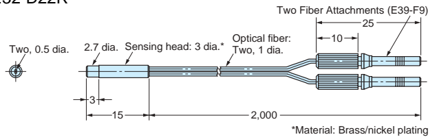
E32-D22 E32-D22R
