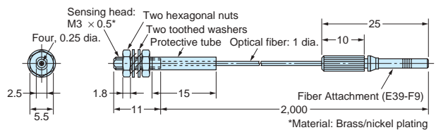
E32-T221B
